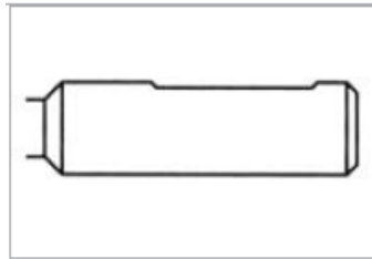
Válcová stopka s čelní plochou - Pro velké průměry (mezi 6-20 mm) - Pro vrtáky s vývrtem pro chladicí prostředek - Zamezuje vytažení vrtáku ze sklíčidla
